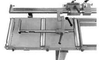
Rollenbahn
